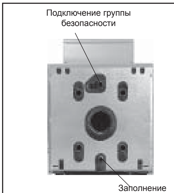
Рис.: Заполнение системы отопления
