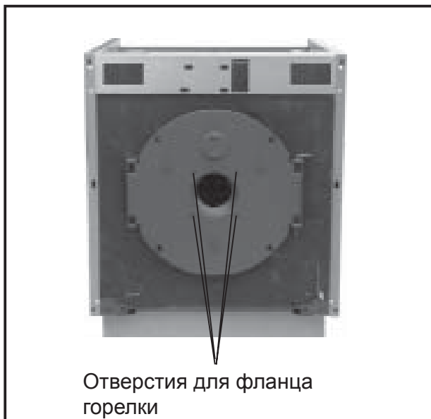
Рис.: Фланец котла
