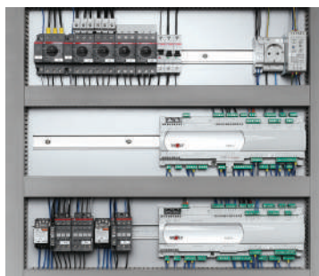
Интегрированный коммутационный шкаф WRS-K компании «Wolf»
