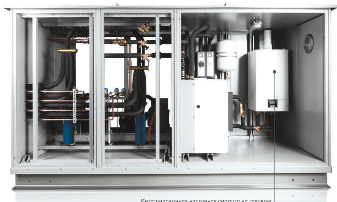
Интегрированная настенная система на газовом отоплении CGB-2 с самой современной техникой использования теплоты сгорания топлива mit modernster Brennwerttechnik für Spitzenlasten
