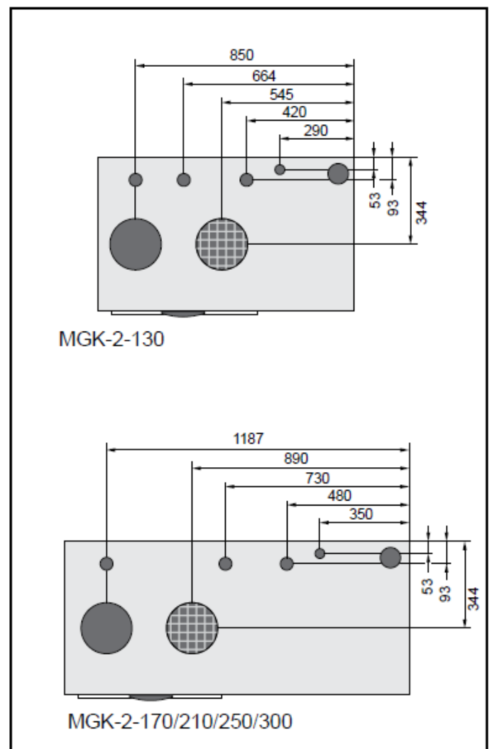
Присоединительные размеры
