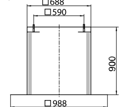
ZBS 09-0071-# Наклонный крышный цоколь
