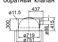
ZLK 21-0710 Моторизированный обратный клапан
