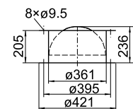
Ручной обратный клапан
