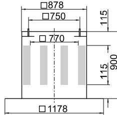
ZDS 20-0090 Цокольный шумоглушитель
