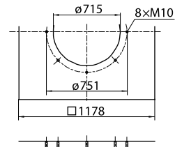
ZBU 01-0090-71 Фланец присоединения
