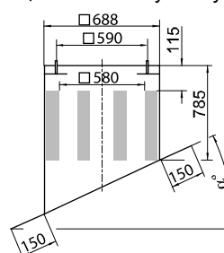
ZDS 09-0071-# Наклонный крышный цокольный шумоглушитель
