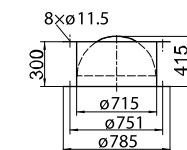
Ручной обратный клапан
