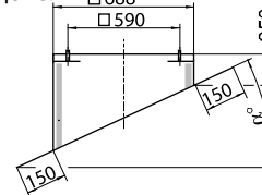
ZBS 09-0071-# Наклонный крышный цоколь
