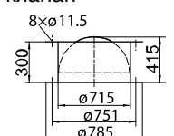
ZLK 01-0710 Ручной обратный клапан
