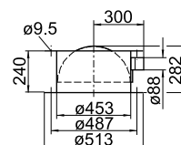
ZLK 21-0450 Моторизированный обратный клапан
