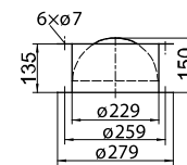
ZLK 03-0225 Ручной обратный клапан
