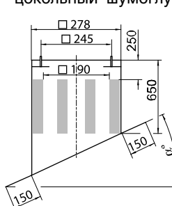
Наклонный крышный цокольный шумоглушитель
