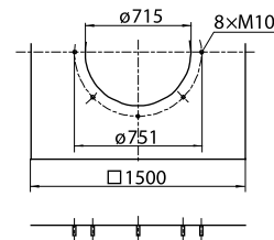
Фланец присоединения
