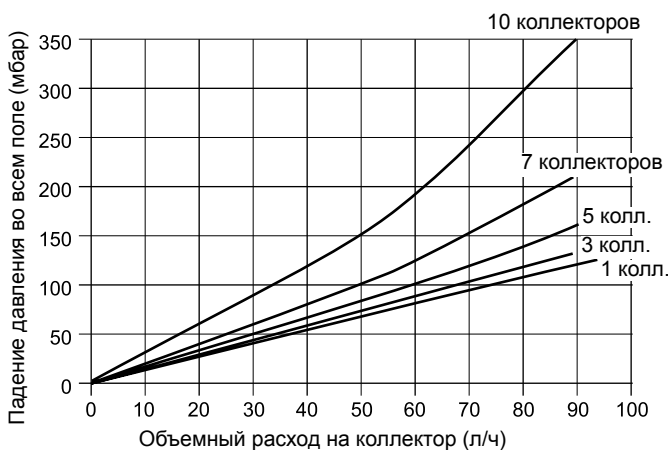
Падение давления F3-1Q с ANRO 30°C
