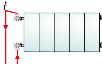
Односторонняя трубопроводная обвязка, слева (возможно до 5 коллекторов)
