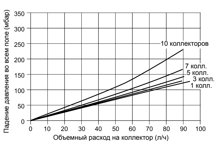
Падение давления F3-1 с ANRO 30°C
