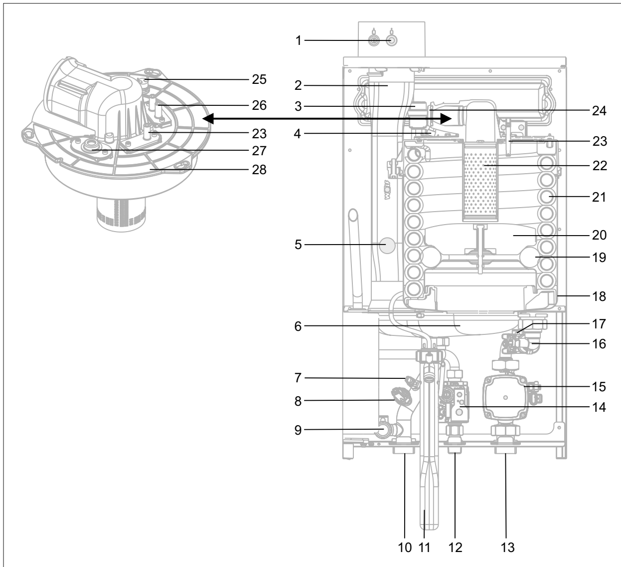
Рис. 3.1 Схема конструкции CGB-2-38 / 55
